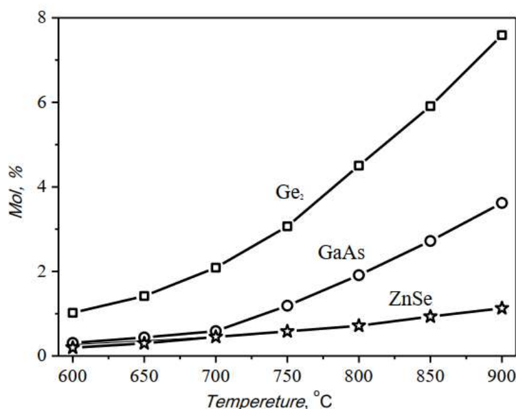
1- rasm. \text{Ge}_2 , GaAs va ZnSe ning Bi dagi eruvchanligining haroratga bog'liqligi.
